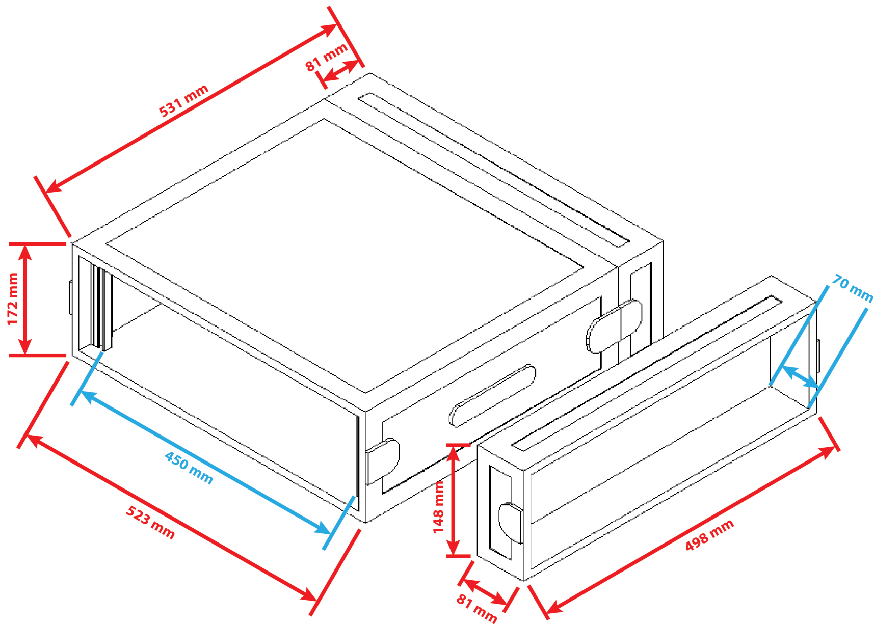
Case 3U Double Door Profi
