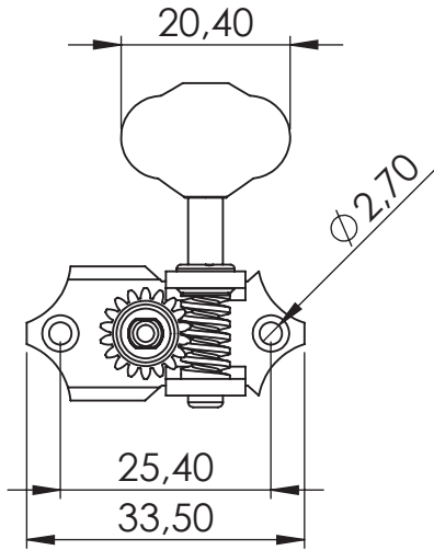
Vorderansicht front view
