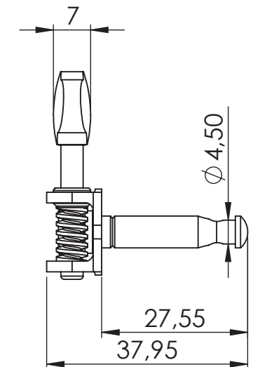
Seitenansicht von rechts side view rechts
