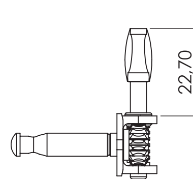
Seitenansicht von links side view left
