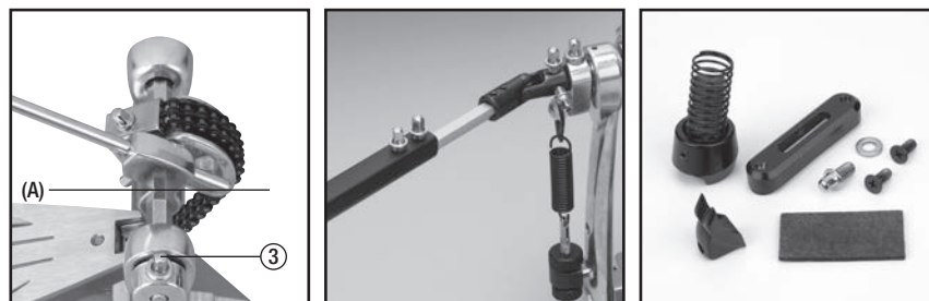
Photo.3 Attaching the Connecting Rod コネクティング・ロッドの取り付け
