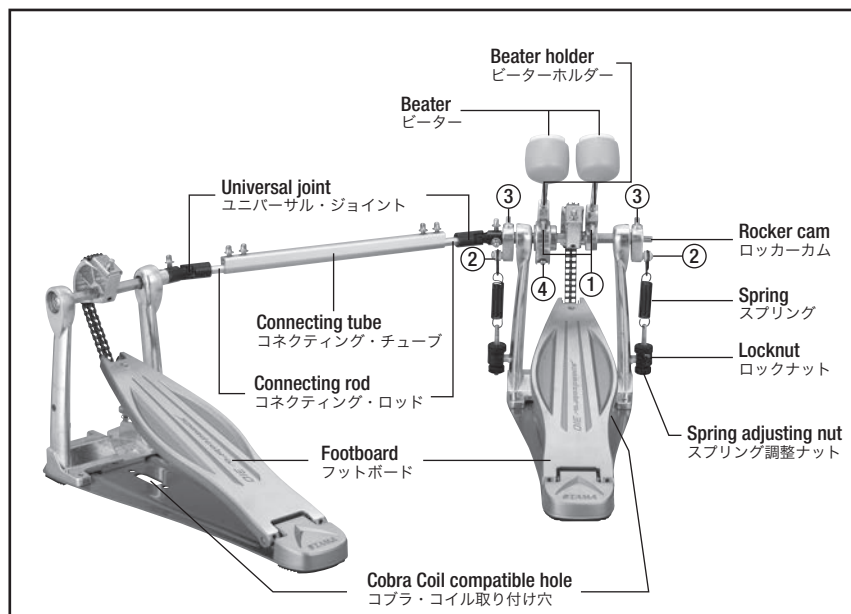
Photo.2 : HP310LW
