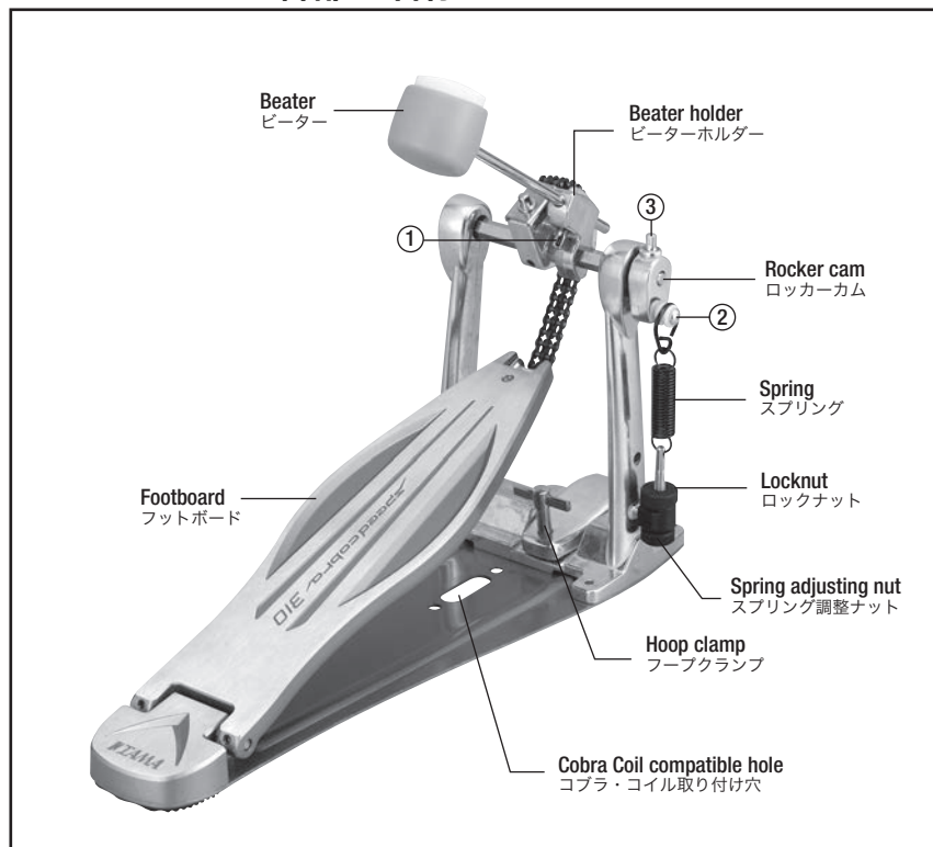
Photo.1 : HP310L
