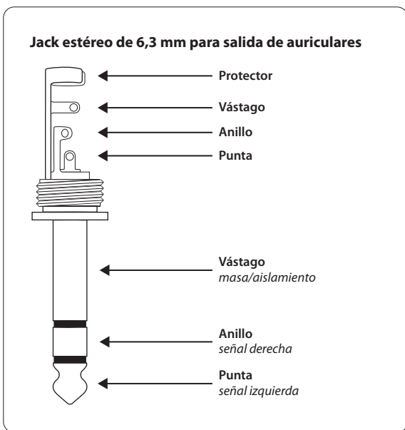
Fig. 3.4: Jack macho estéreo para auriculares
