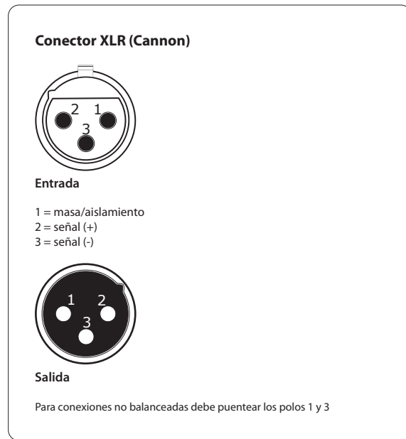
Fig. 3.1: Conexiones XLR
